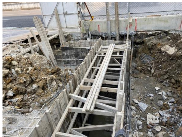
導溝施工
