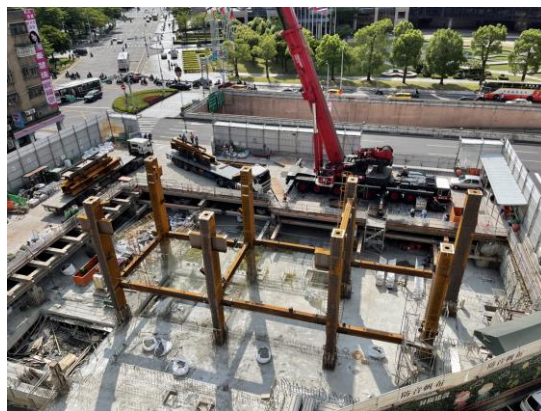
鋼柱吊裝
