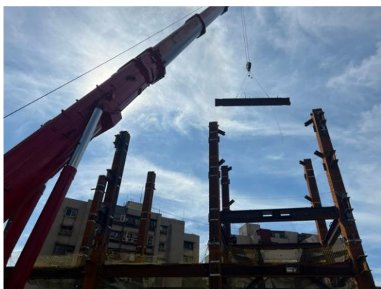
鋼梁吊裝
