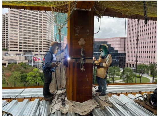
鋼柱對焊
