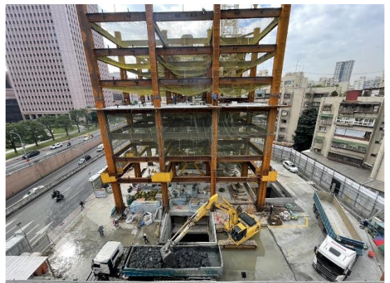
鋼構第三節完成
