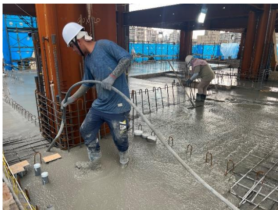
混凝土搗築
