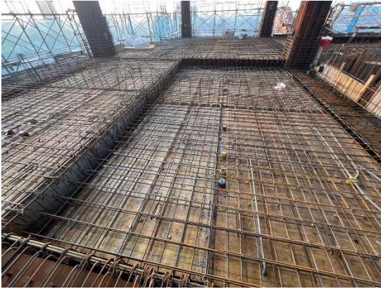
版筋綁紮
