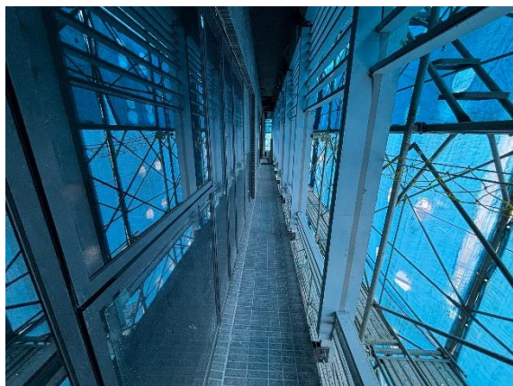
外牆磁磚及金屬隔柵施作
