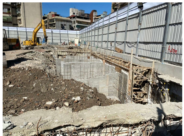
深導溝施工
