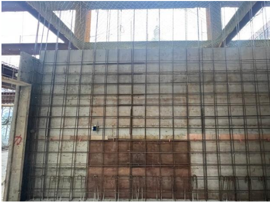
牆筋綁紮
